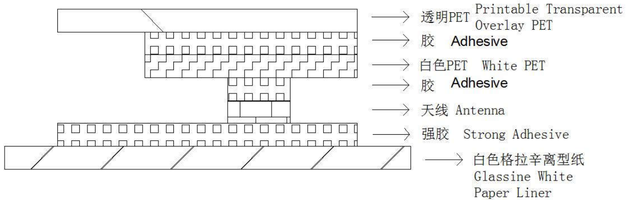
标签结构图 Label Layer Structure
